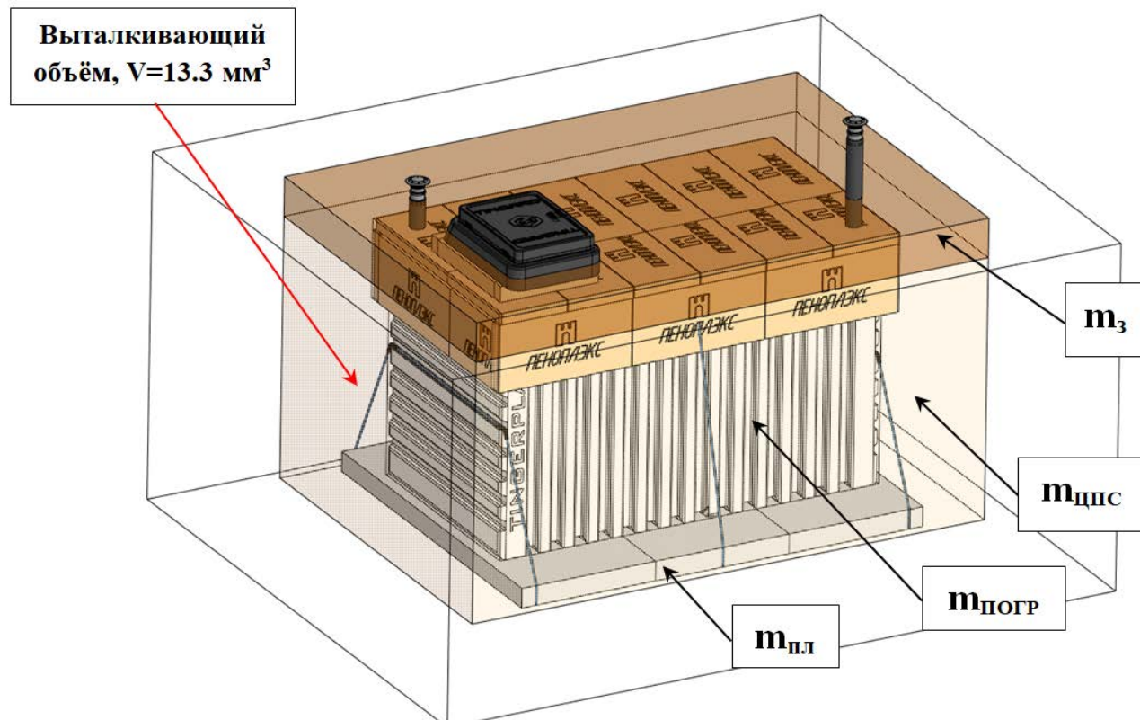
Рисунок 11 – Расчет якорения погреба
